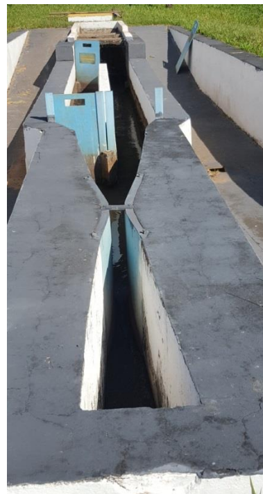
Foto 3.11 - Calha Parshall e Caixa de Areia – Entrada ETE
