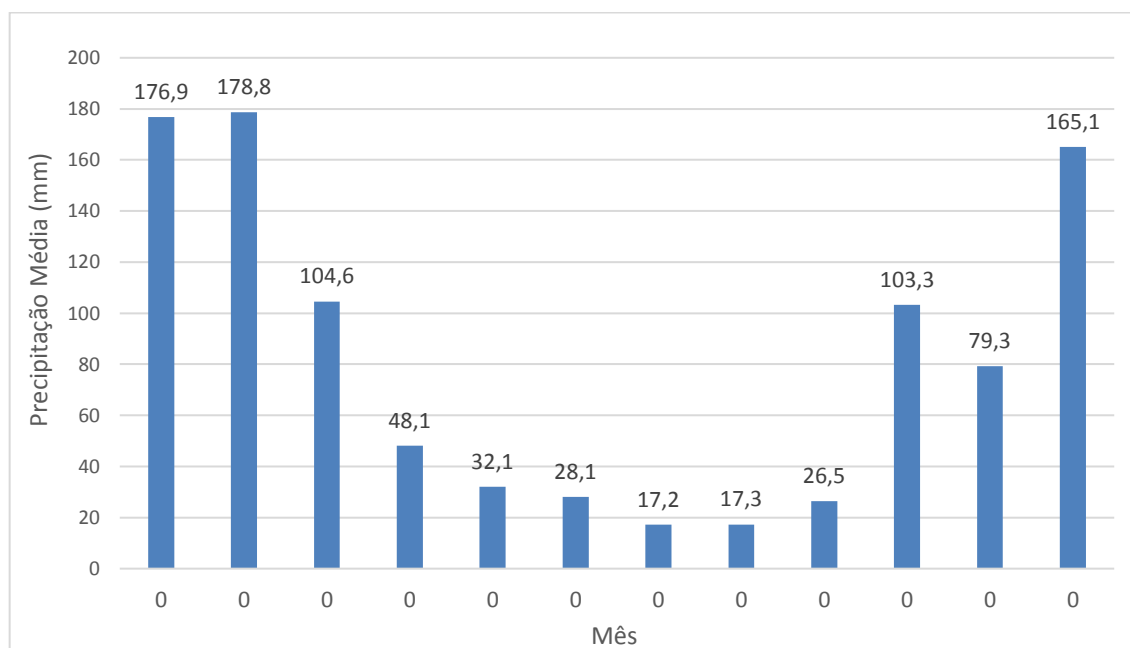
Gráfico 2.1 - Precipitação Média Mensal no Período de 1959 a 1971, Estação B7-003
